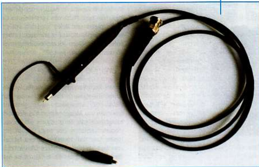
Figuur 2. 1:1 / 10:1 meetprobe
